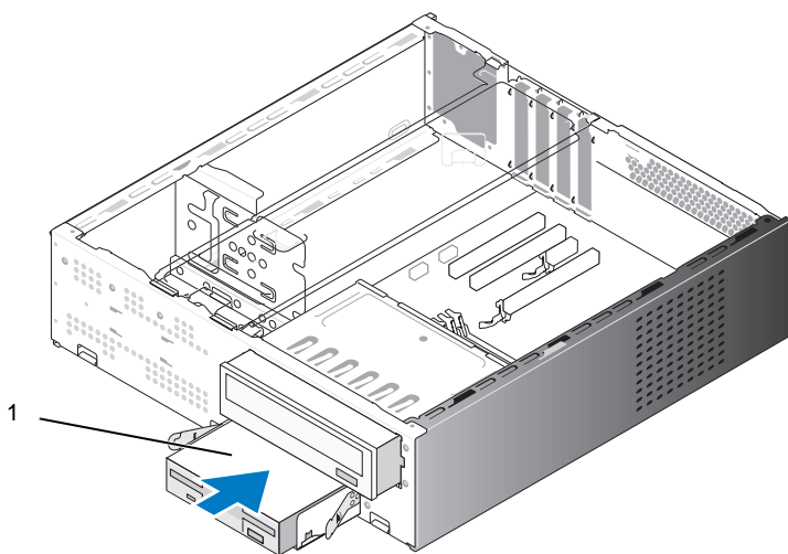
1 дисковод гибких дисков
