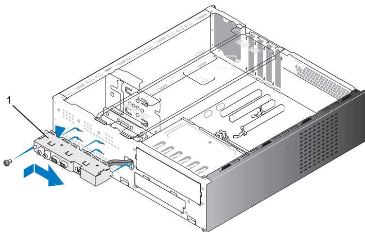
1 панель ввода/вывода
